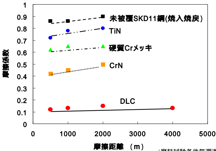
各種硬質皮膜の摩擦係数
