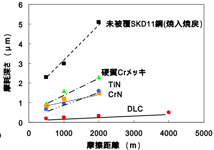
各種硬質皮膜の摩耗深さ
